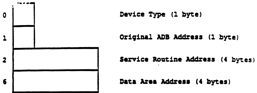
Figure 5. ADB Data Parameter Block
