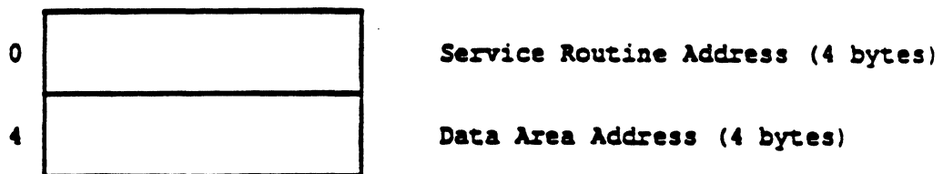
Figure 6. SetInfo Parameter Block
