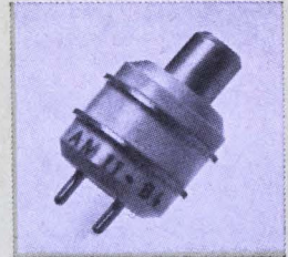
Actual size GE Y-1537 planar ceramic triode
